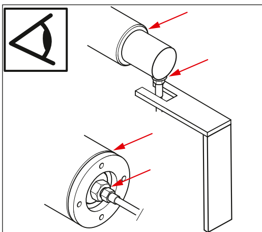
Abb. 8: Sichtkontrolle ausführen
